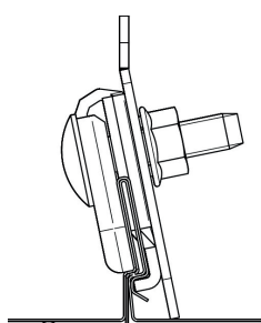
Kuva 4. LE-kiinnike ja vastarauta kiristettynä saumaan
