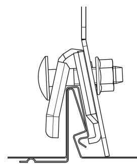
Kuva 3. LE-kiinnike ja vastarauta asemointi ponttiin
