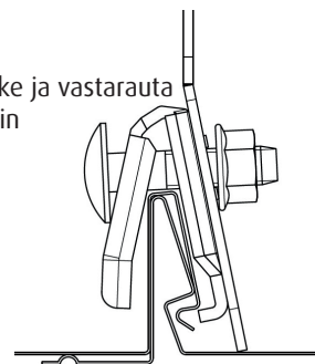
Kuva 6. Osaluettelo sekä vastaraudan aseointi.
