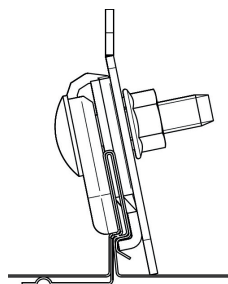
Kuva 5. LE-kiinnike ja vastarauta kiristettynä saumaan
