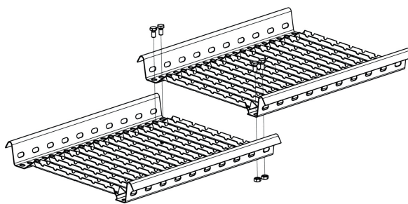
Kuva 8. Kattosillan jatkaminen
