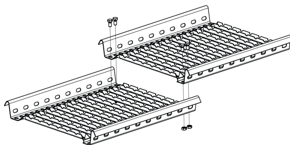
Kuva 8. Kattosillan jatkaminen
