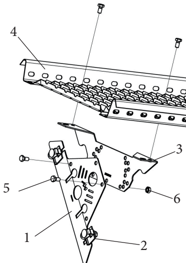
Kuva 6. Osaluettelo sekä vastaraudan asemointi.
