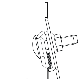
Kuva 5. Le-kiinnike ja vastarauta kiristettynä saumaan
