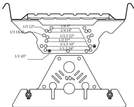
Kuva 7. Yleisimmät kattokaltevuudet
