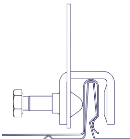
kuva 2 Lukkosaumakate
