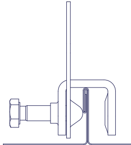
kuva 3 Konesaumakate
