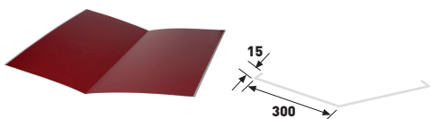
Разжелобка JL
