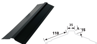
Конёк прямой
