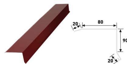
Пристенная планка
