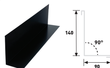
Пристенная планка
